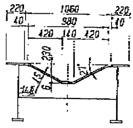
フォルクスワーゲン のトラス(4軸) 700-2000mm
